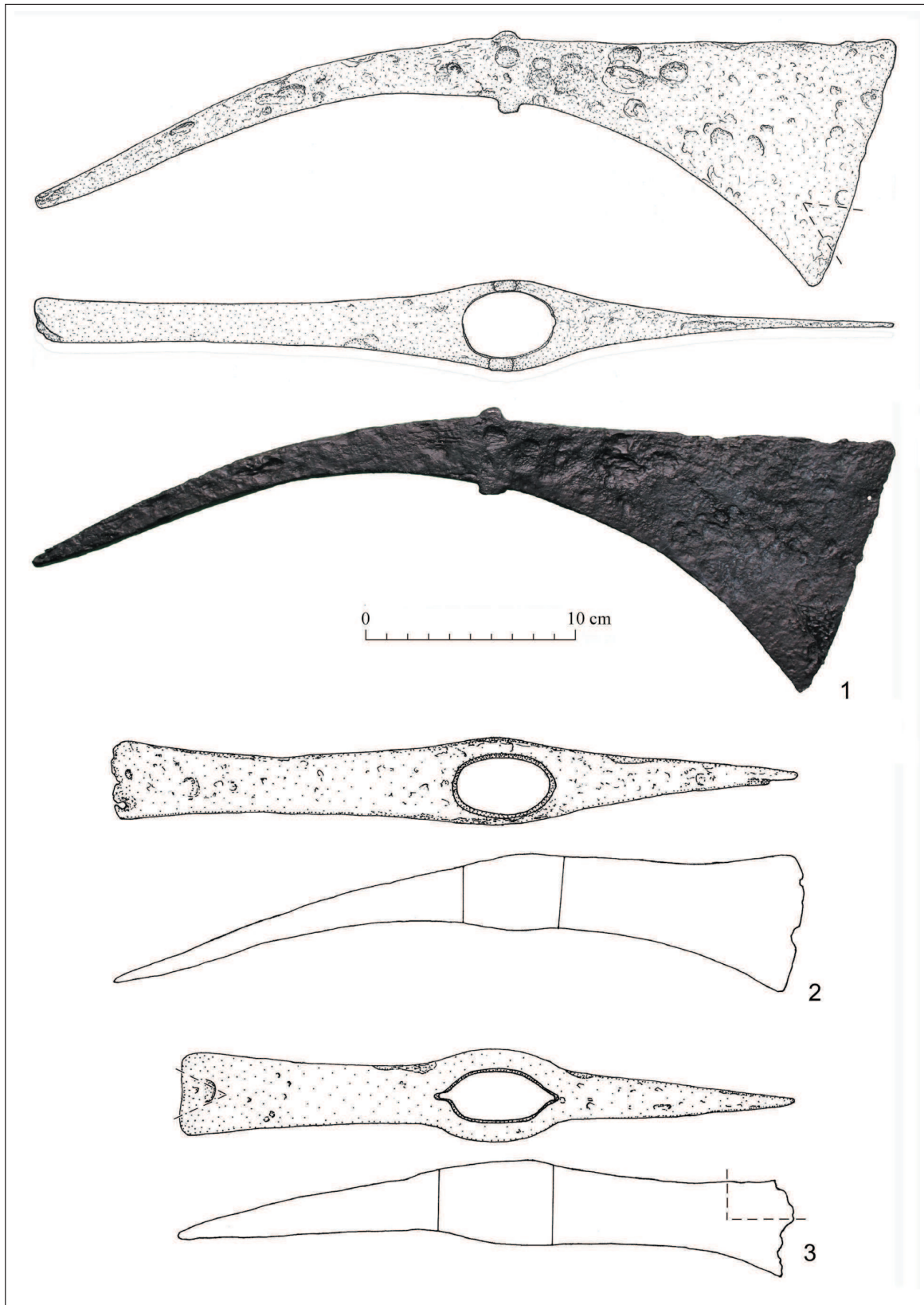
Obr. 2 Rímske dolabrae z územia Slovenska: 1 koryto Dunaja, 2,3 Dunajská Lužná (miesta odberu vzoriek na metalografické analýzy vyznačené prerušovanou líniou). Abb. 2 Römische Dolabrae aus dem Gebiet der Slowakei: 1 Flussbett der Donau, 2,3 Dunajská Lužná (Stellen der Musterziehung für metallgraphische Analysen sind mit einer unterbrochenen Linie markiert).
