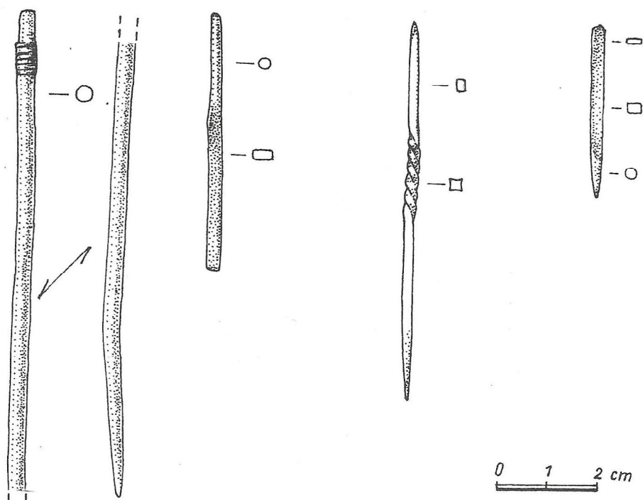
Obr. 11. Dedinka - čakanská osada. Bronzový inventár sídliskového objektu III/80
