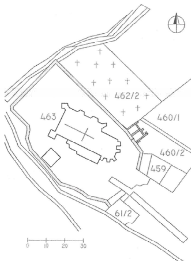
Obr. 1 Svätý Jur. Situačný plán Kostola sv. Juraja s okolím; M 1 : 500
